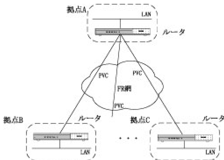
ツリー型のネットワーク構築例
