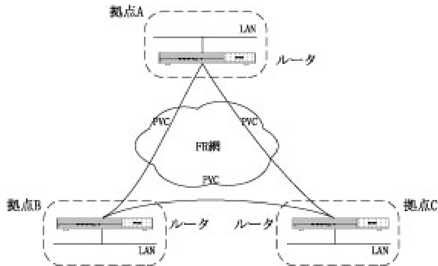
メッシュ型のネットワーク構築例
