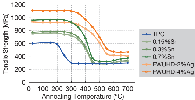
【軟化特性・耐熱性】 Thermal resistance at \phi 0.06 \text{ mm}
