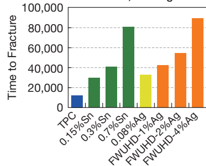
【耐屈曲性】 Bending fatigue at \phi 0.06 \text{ mm} r=10 \text{ d, W}=20 \text{ g}
