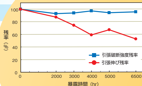
パイプ本体外層材の引張試験結果
