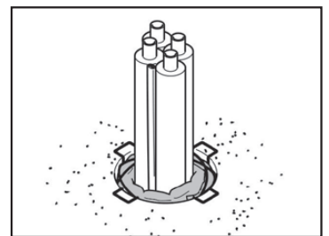
イチジカン-耐火パック
