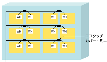
集合住宅：幹線横引き
