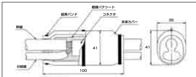
エフタッチカバー・ミニ 寸法
