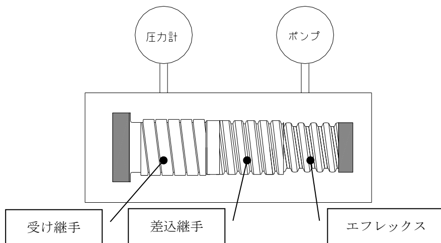
図－ 3 水密試験
