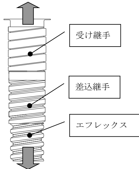
図－４ 引張試験
