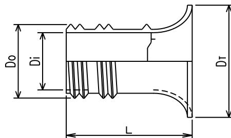
図－１ 構造
