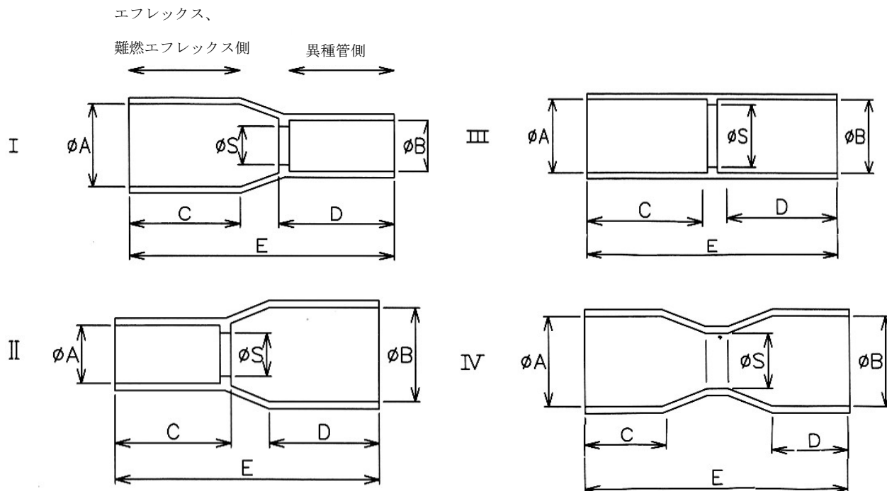
図－2 構造図
