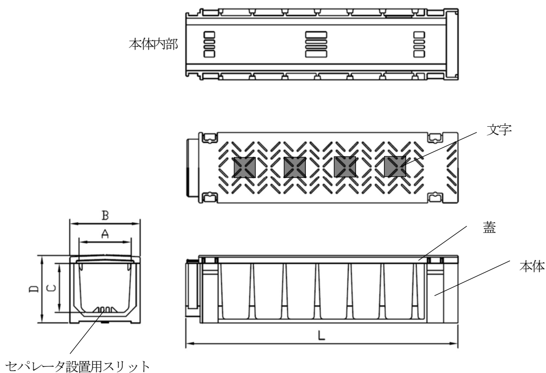
付図2 直管 複孔式 文字入り蓋
