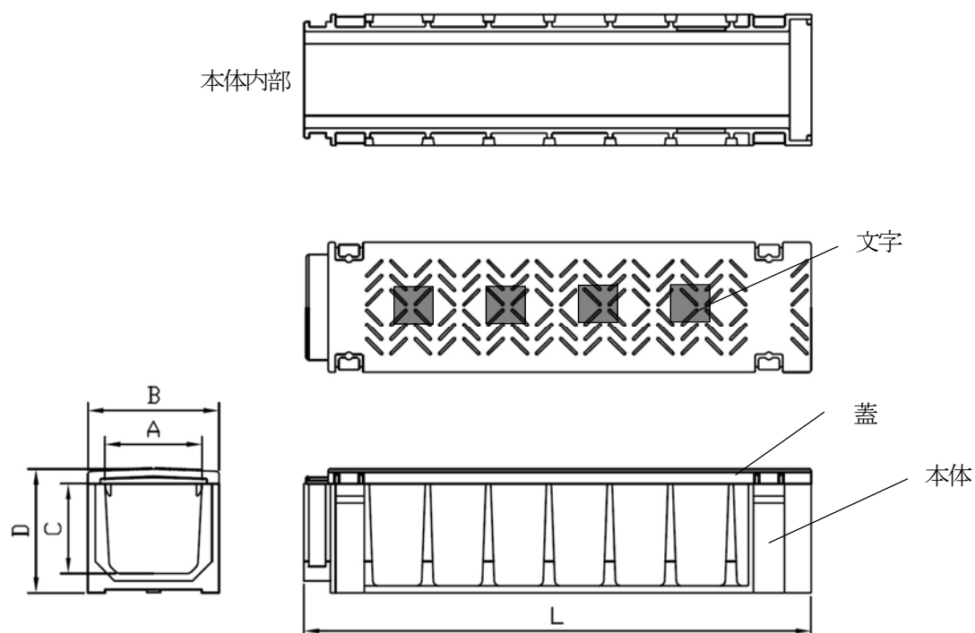
付図1 直管 文字入り蓋
