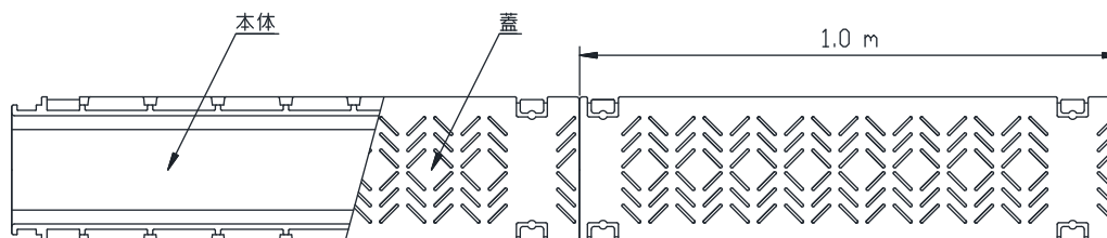
図－1 構造（120S,150S, 200B,300B,300C 組図）
