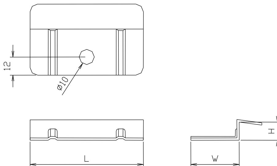
付図 1 9 ズレ防止金具
