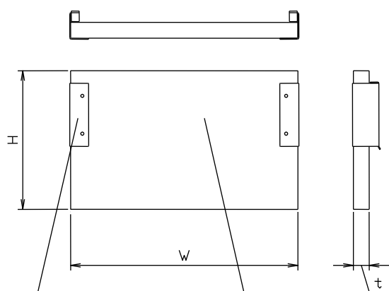
付図 1 1 端面板
