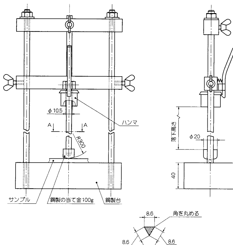
図-4 衝撃試験装置
