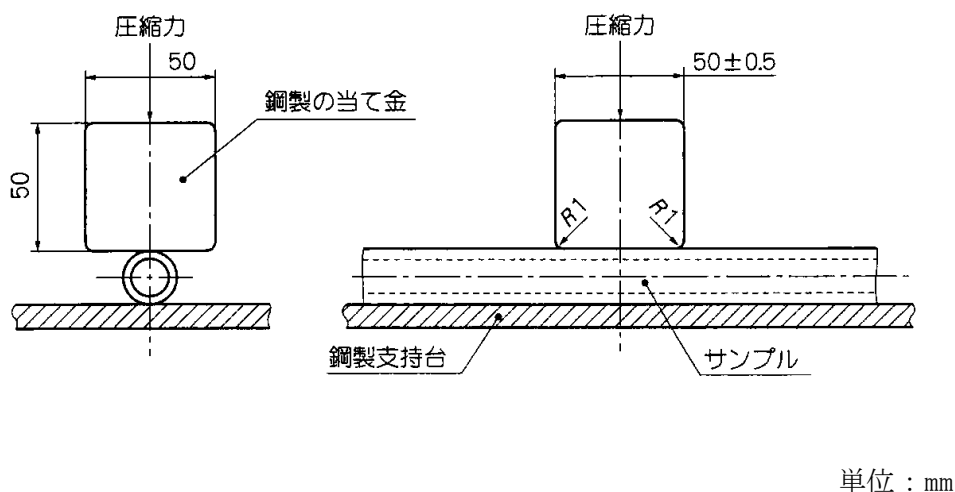
図 3 圧縮試験の配置
