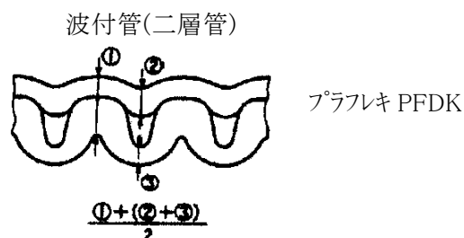
図 6 厚さの測定方法
