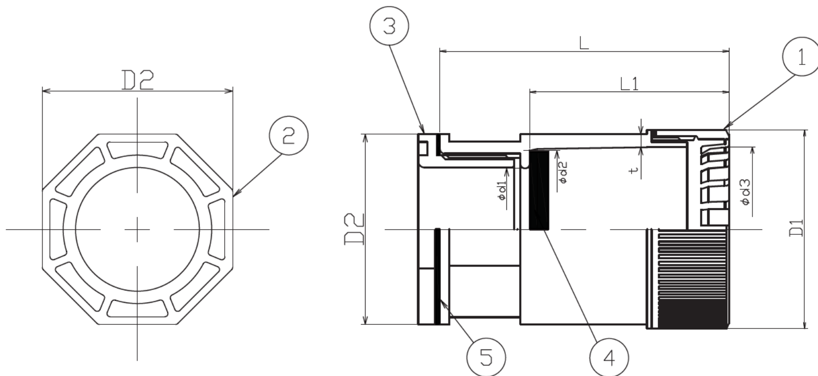
寸法表 単位: mm
