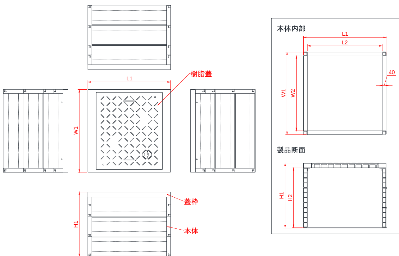
付図2 ROM-Box 組図 750×750 サイズ
