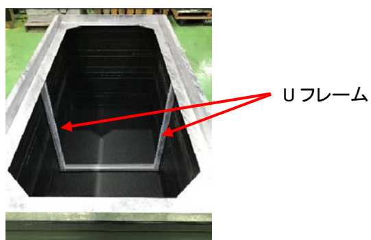
図 5 ROM-Box 750×1550 サイズ内部
