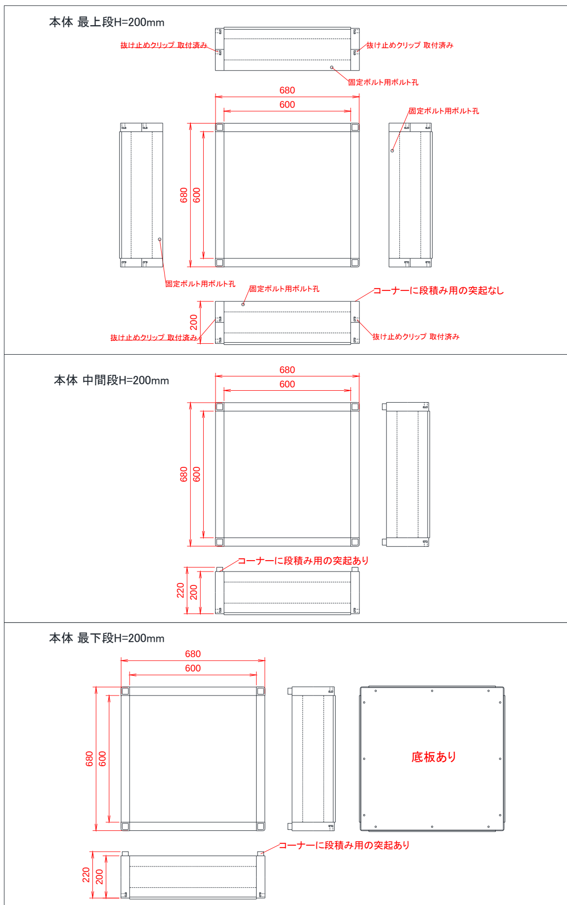
付図 4. 構成部材 参考図 1 (600×600 用 本体)
