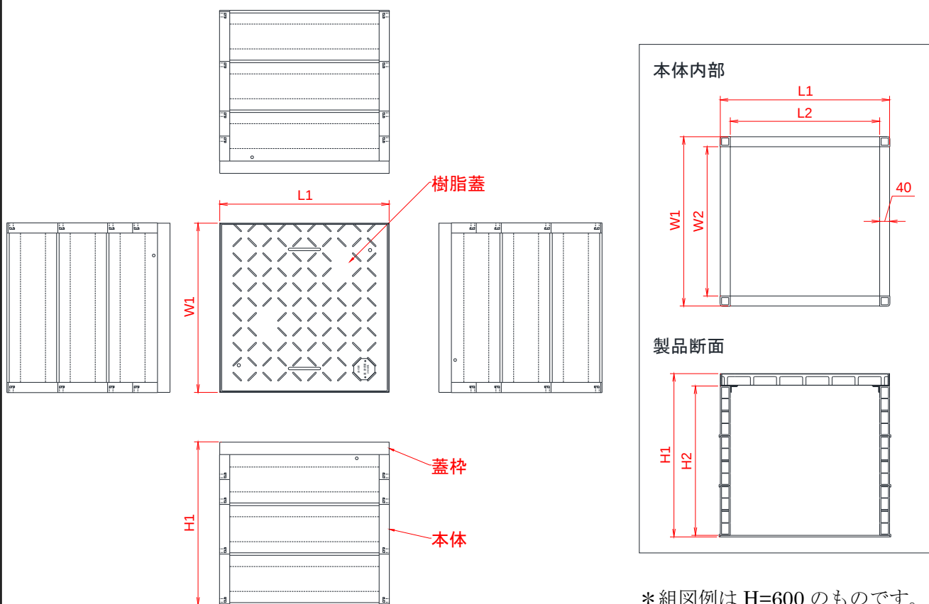
付図1 ROM-Box 組図 600×600 サイズ
