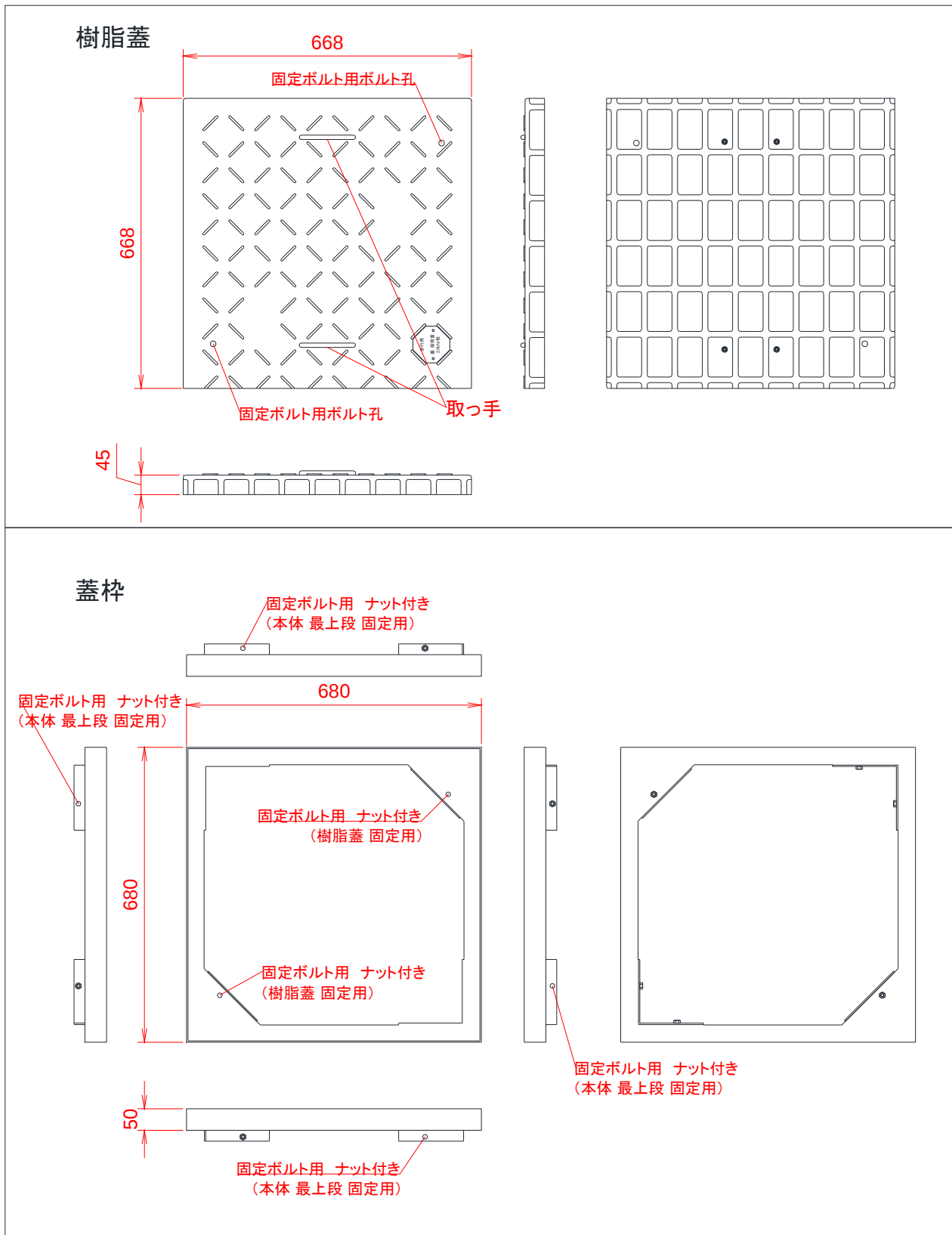
付図 5. 構成部材 参考図 2 (600×600 用 樹脂蓋、蓋枠)
