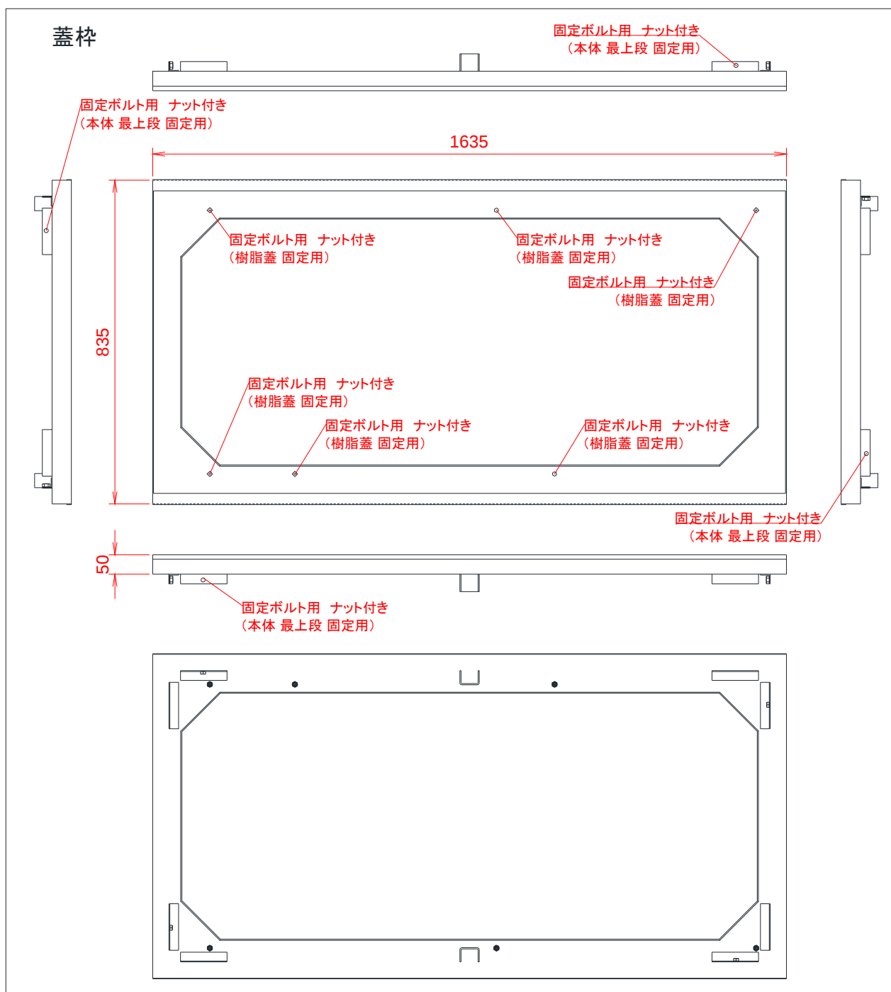
付図 10. 構成部材 参考図 7 (750×1550 用 蓋枠)
