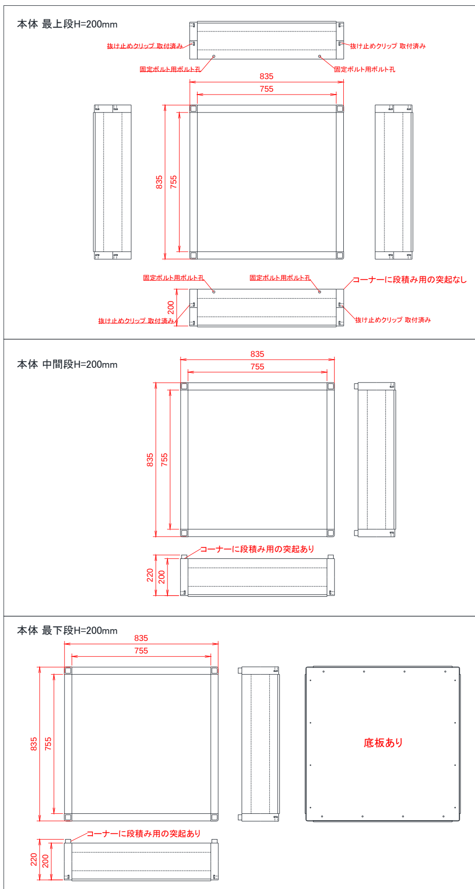
付図 6. 構成部材 参考図 3 (750×750 用 本体)
