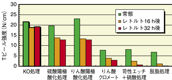
図4 各種処理材のエポキシ接着剤に対するTピール強度 T-peel strength of the KO and other surface treatments for epoxy bond.
