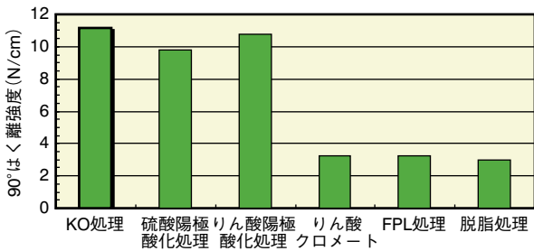
図3 各種処理材のアクリル系粘着剤テープに対する90°はく離強度 90 peeling strength of KO and other surface treatments for acrylic adhesives.
