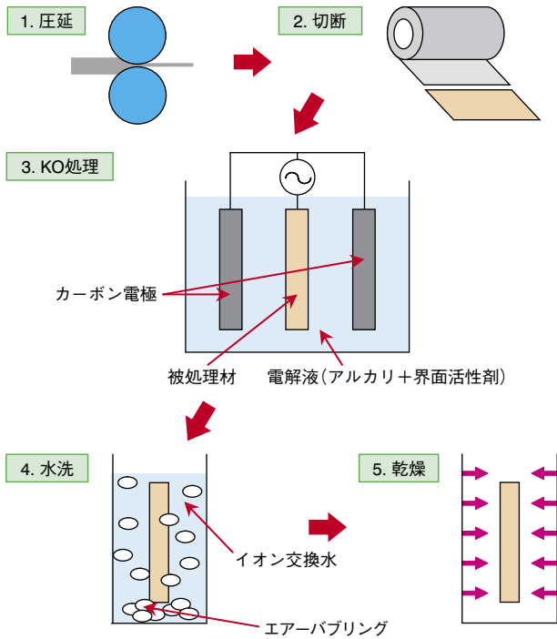
図2 KO処理 KO process.
