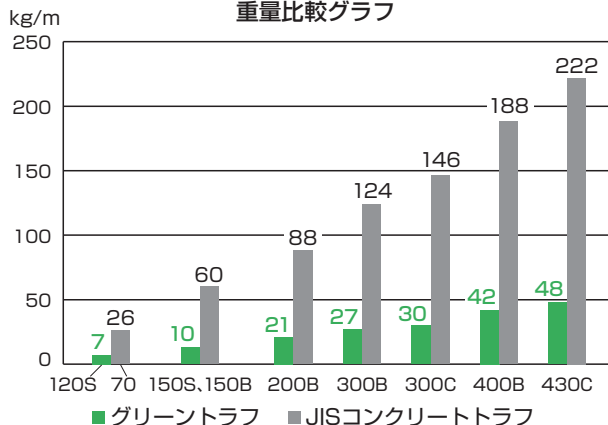
グリーントラフ vs JISコンクリートトラフ 重量比較グラフ
