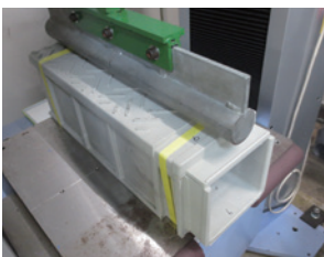
耐荷重試験の様子
