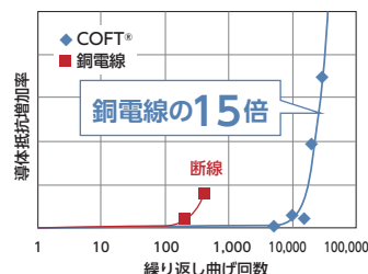
繰り返し曲げによる導体抵抗増加率
