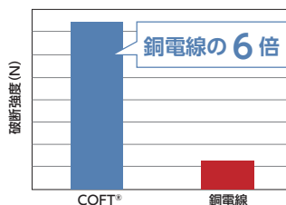
引張り試験による破断強度
