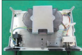
スプリッタプレ配線例 ※2
