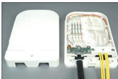
融着接続
