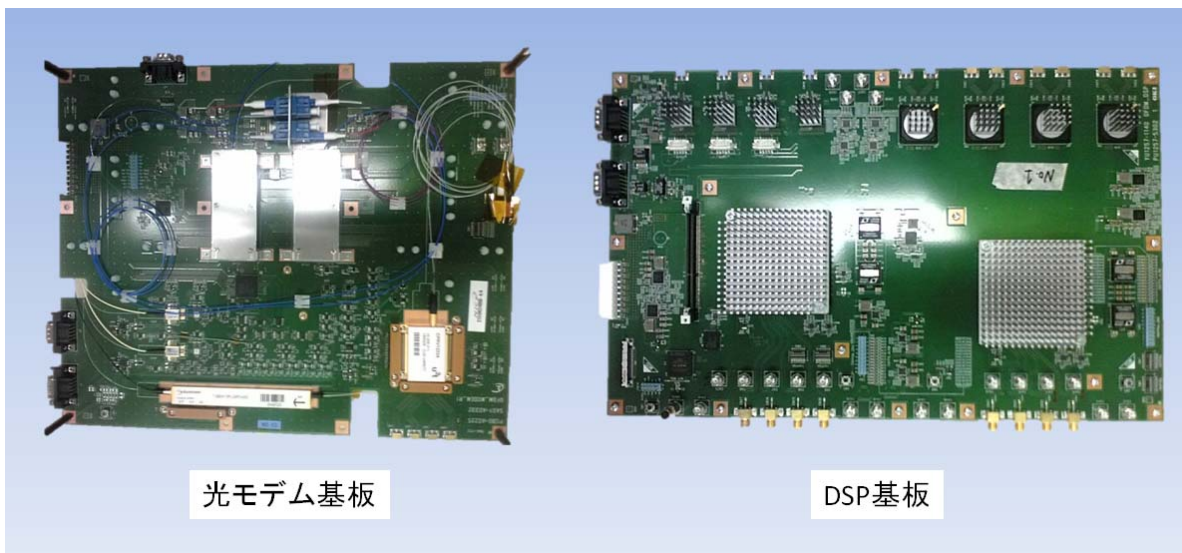
図4 開発した適応変復調 OFDM 伝送方式対応光送受信器の写真(OKI)
